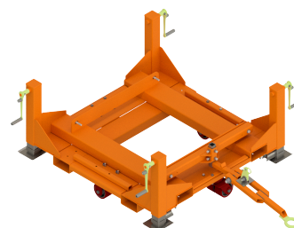
Base du cube + Stabilisateur du cube
